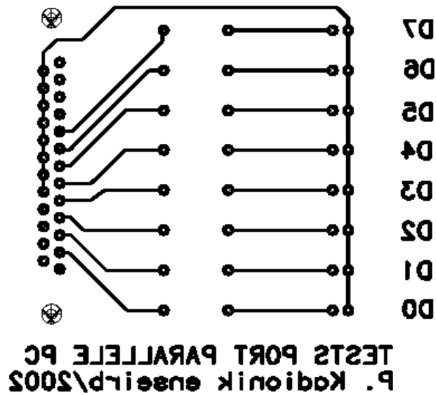
Figure 8 : typon du module électronique
