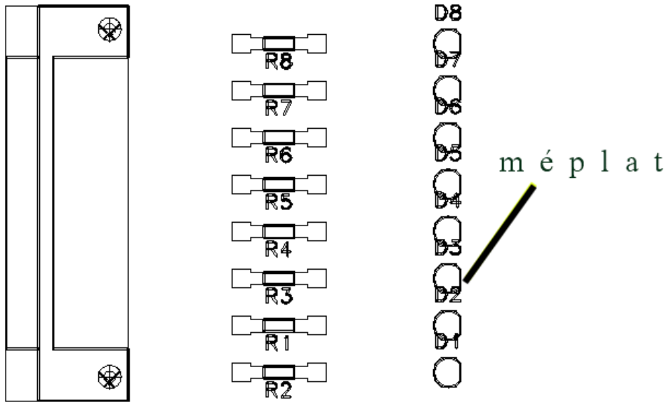
Figure 9 : layout du module électronique
