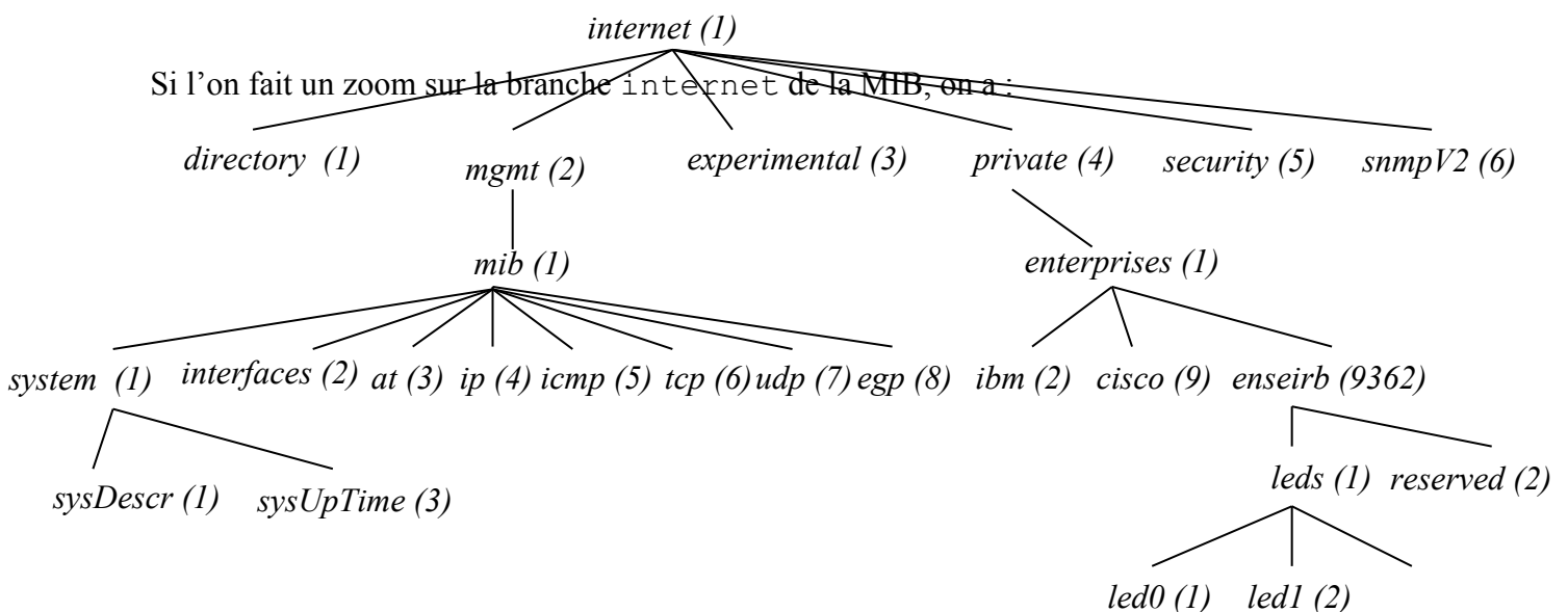
Figure 5 : structure de la MIB
