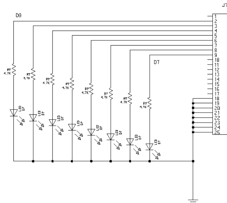
Figure 7 : schéma électrique du module électronique
